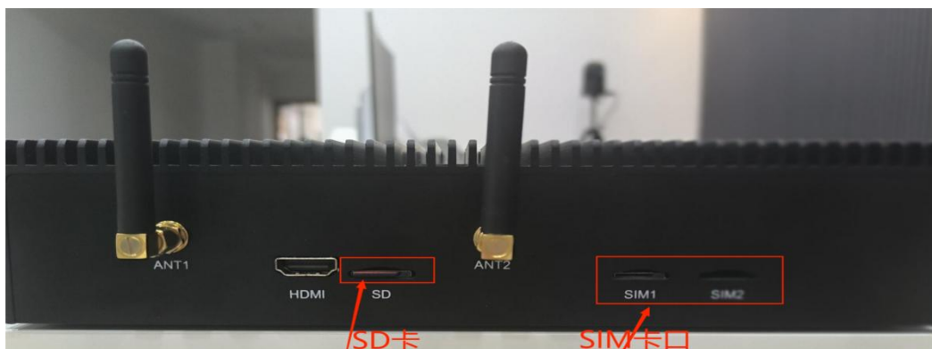
图3 正面图
